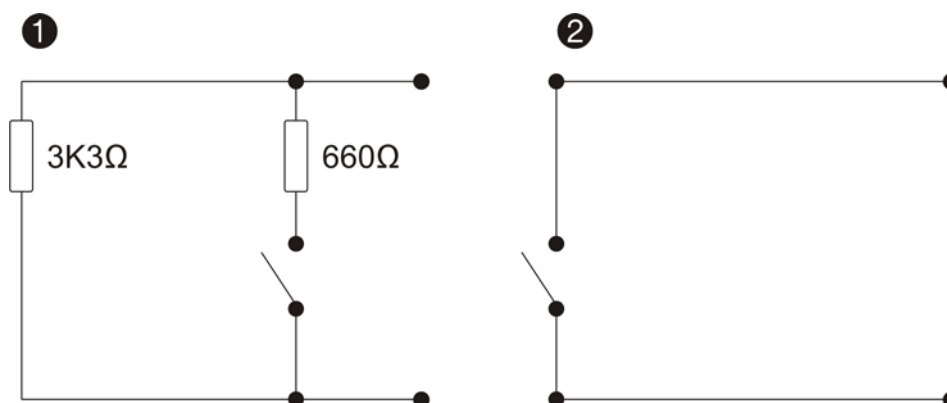
Rysunek 8: Opcje konfiguracji zworek
