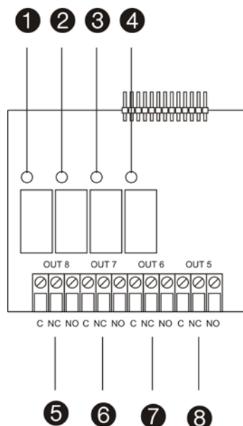
Rysunek 6: Wspólny moduł we./wy. – przekaźniki z możliwością programowania
